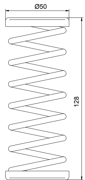
(4) Muelle exterior
